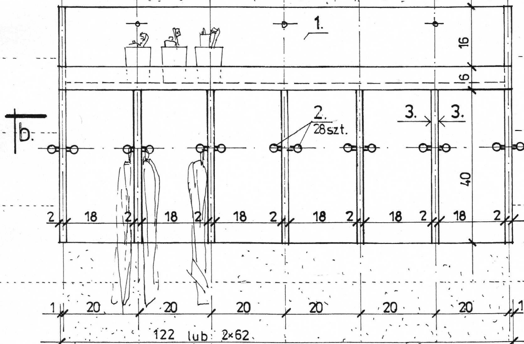
WIDOK 1:10
