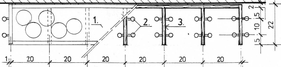
RZUT
