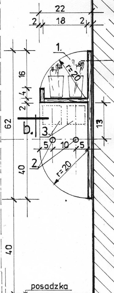
PRZEKRÓJ a-a 1:10
